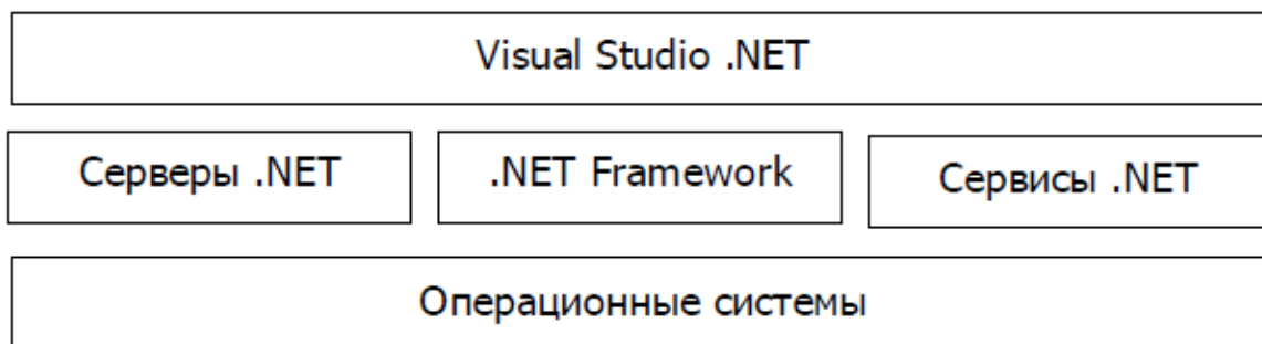
Рисунок 1 Платформа Microsoft.NET
