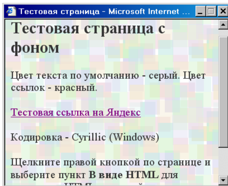
Рис. 4. Пример страницы
