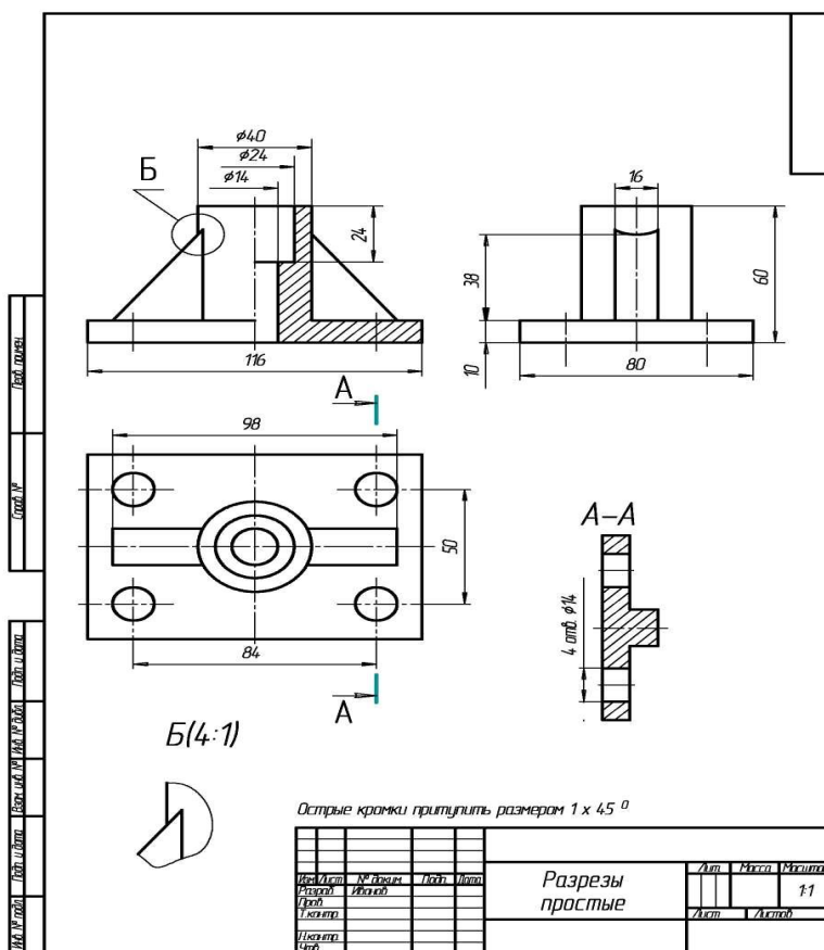
Рис. 3.22. - Пример выполнения задания «Разрезы»
