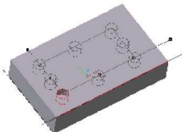
Рис. 7.14. - Фантом массива отверстий в прямоугольной В окне детали отображается фантом массива (рис. 7.14), что позволяет оценить правильность задания параметров и при необходимости внести в них изменения.
