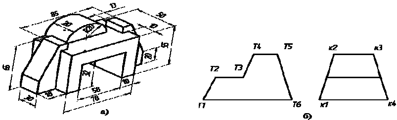
Рис. 1.17. - Исходные данные задания лабораторной работы: а) изометрическая проекция детали; б) комплексный чертеж детали
