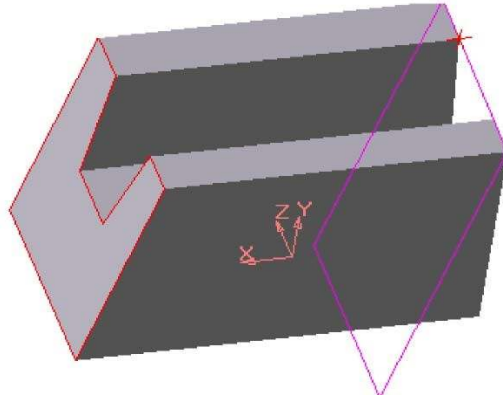
Рис. 6.9. - Вспомогательная плоскость через вершину параллельно боковой грани
