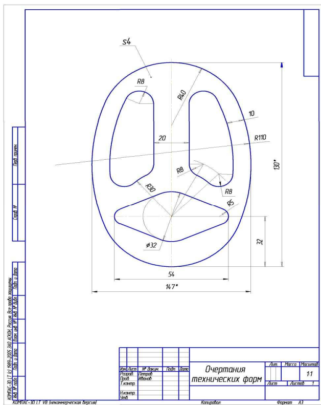
Рис. 2.13 - Пример выполнения работы «Очертание технических форм»
