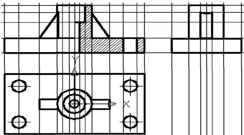
Рис. 3.14. - Использование вспомогательных прямых
