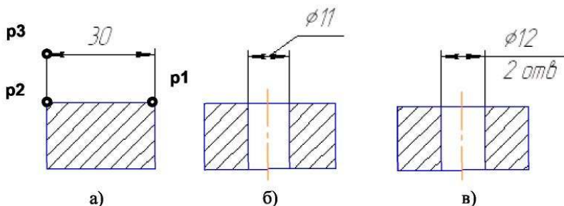
Рис. 2.8. - Варианты нанесение линейных размеров
