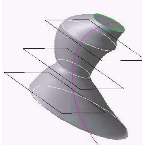
Рис. 5.18. - Модель тела с криволинейной направляющей
