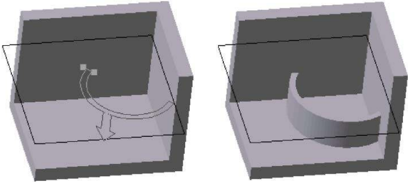
Рис. 7.6. а) модель на этапе формирования ребра жесткости с использованием команды б) модель с выполненным ребром жесткости (Ортогонально плоскости эскиза)
