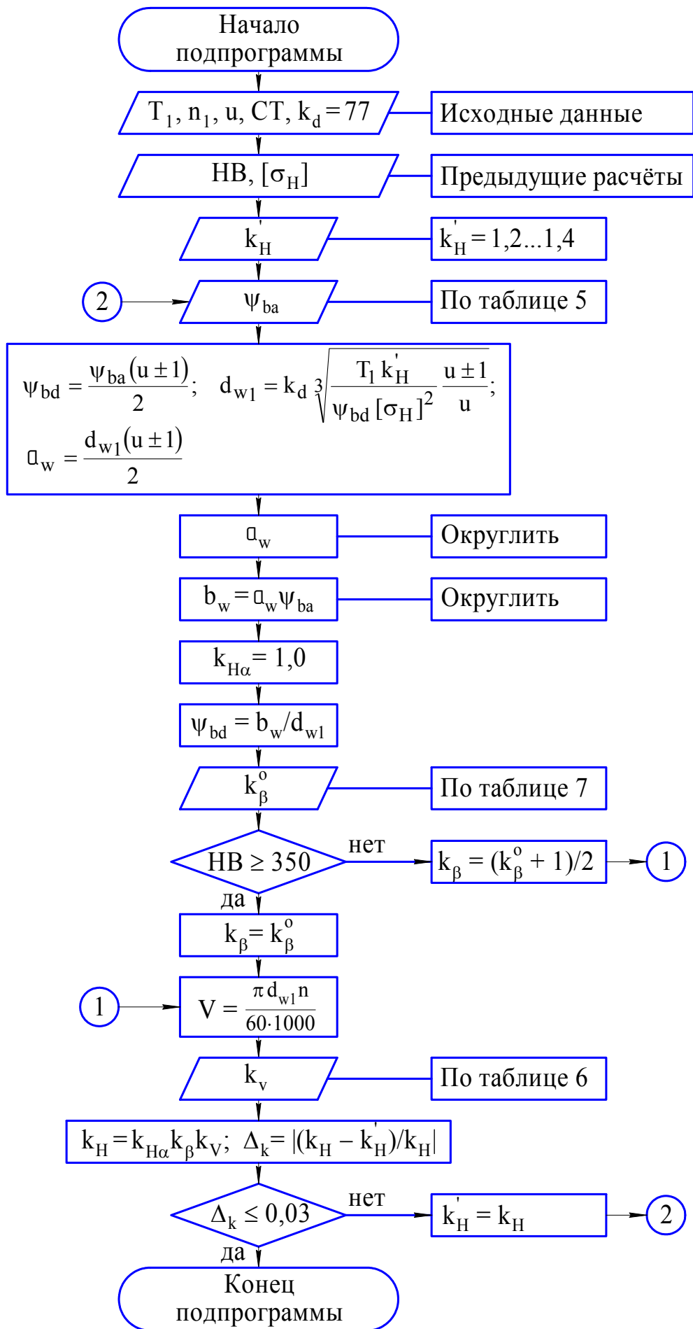
Рис. 10. Схема алгоритма определения габаритов передачи
