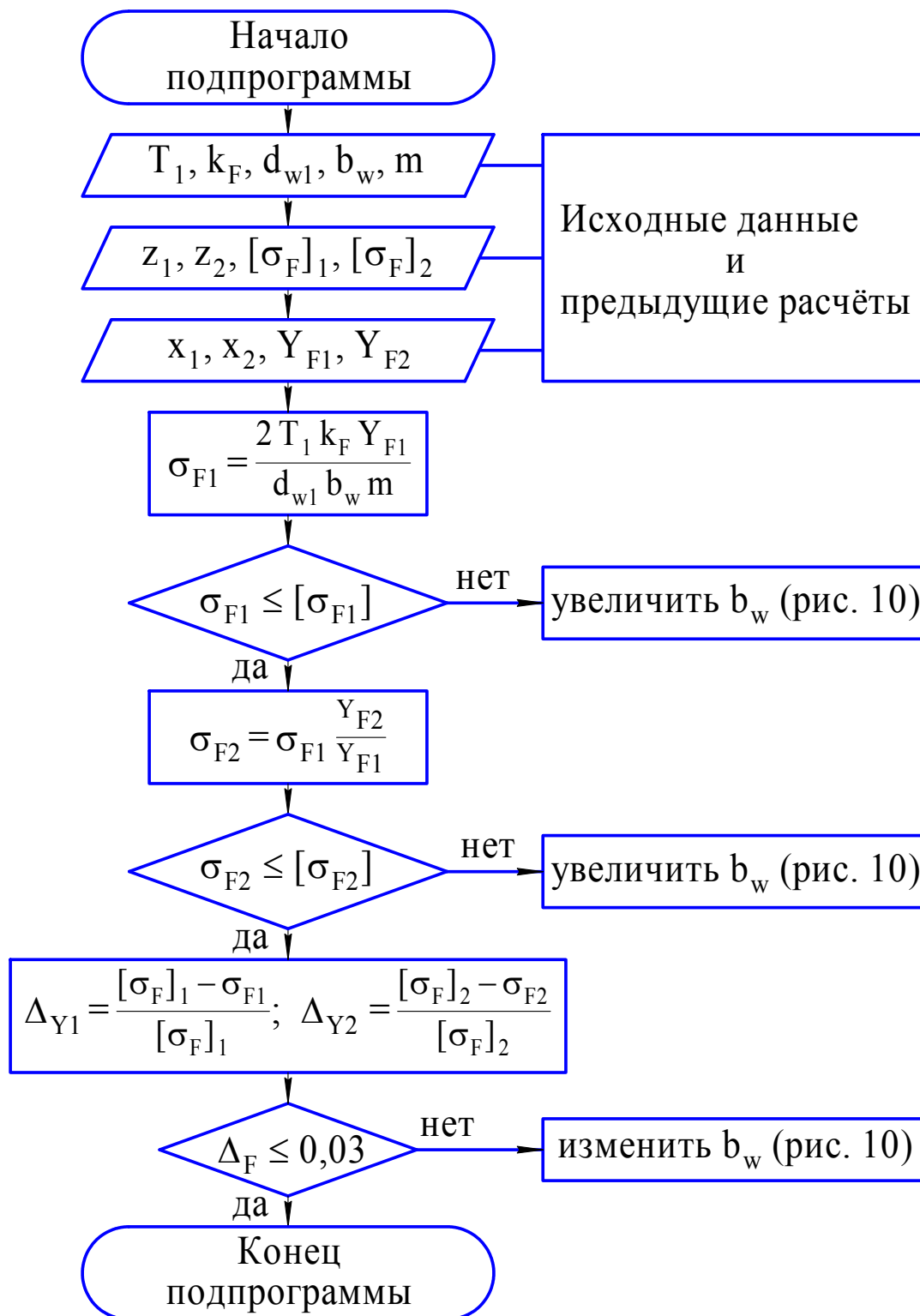
Рис. 17. Схема алгоритма проверки изгибной прочности передачи
