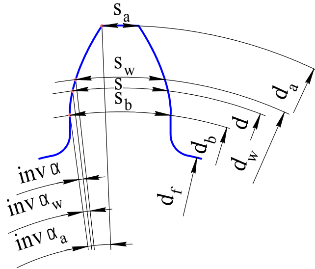
Рис. 14. Геометрические размеры зубчатого колеса
