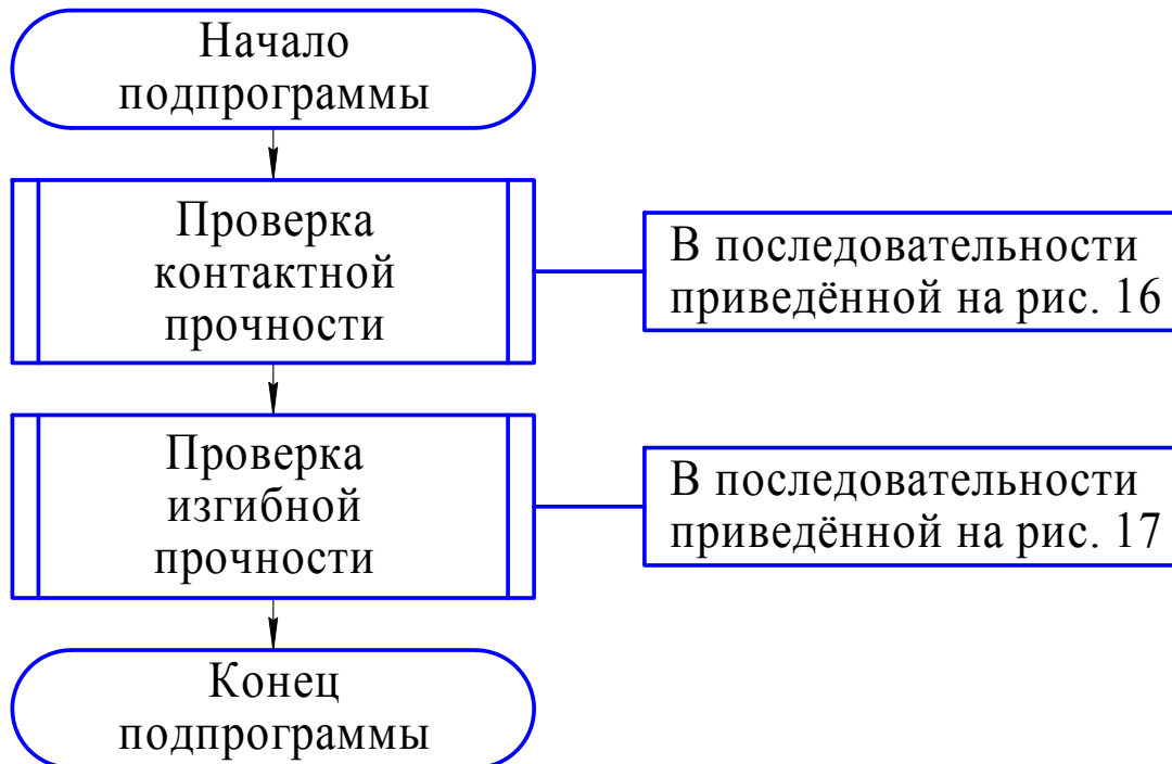
Рис. 15. Схема алгоритма проверки прочности передачи
