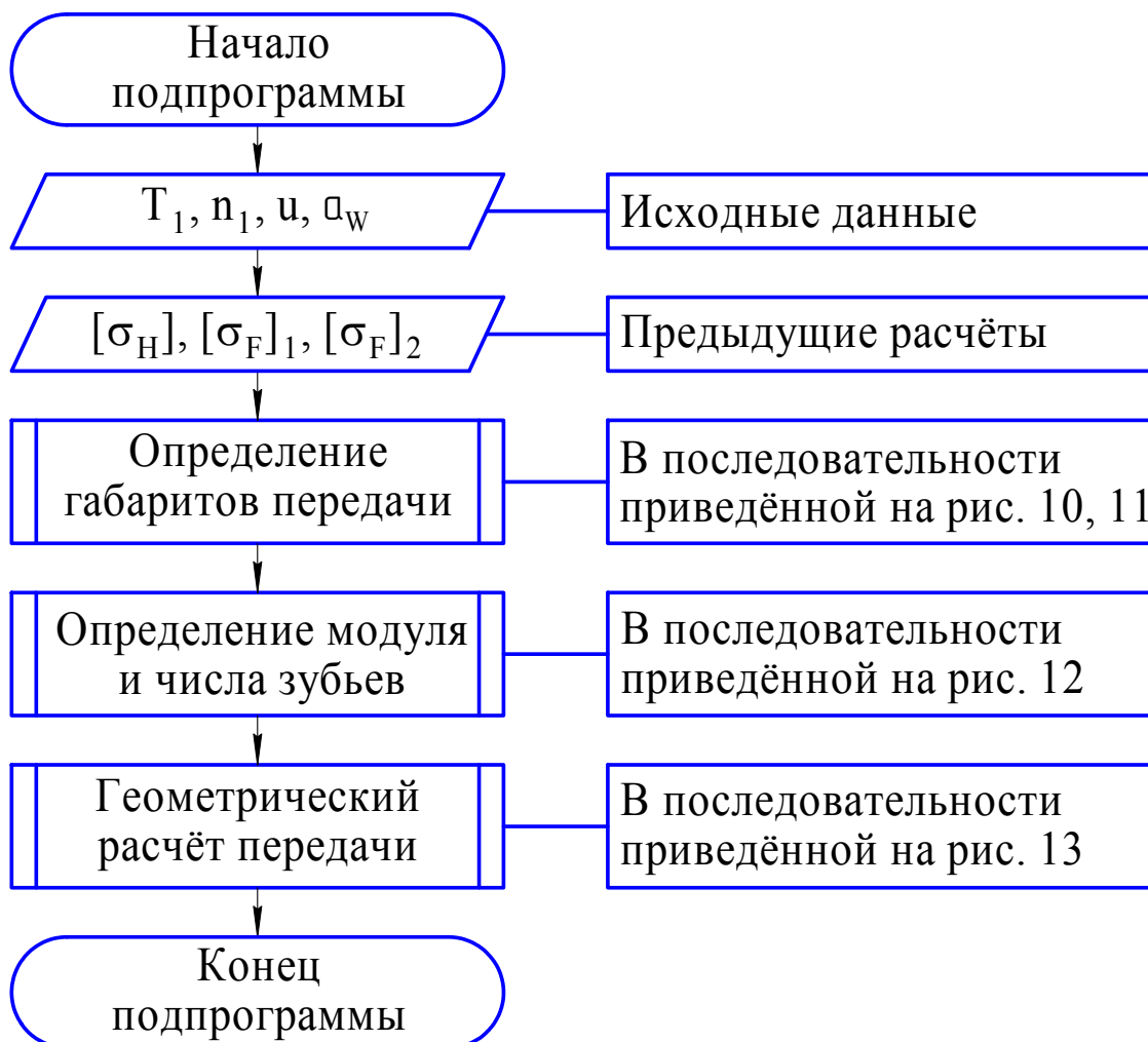
Рис. 9. Общая схема алгоритма определения размеров передачи
