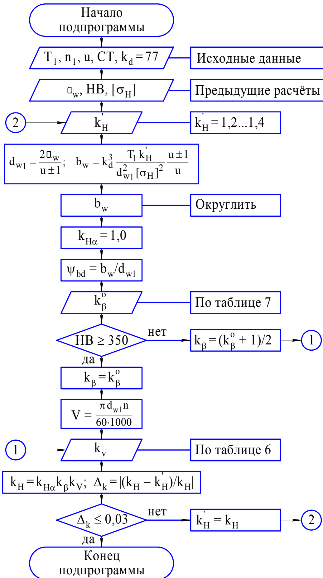
Рис. 11. Схема алгоритма определения габаритов передачи при заданном межосевом расстоянии
