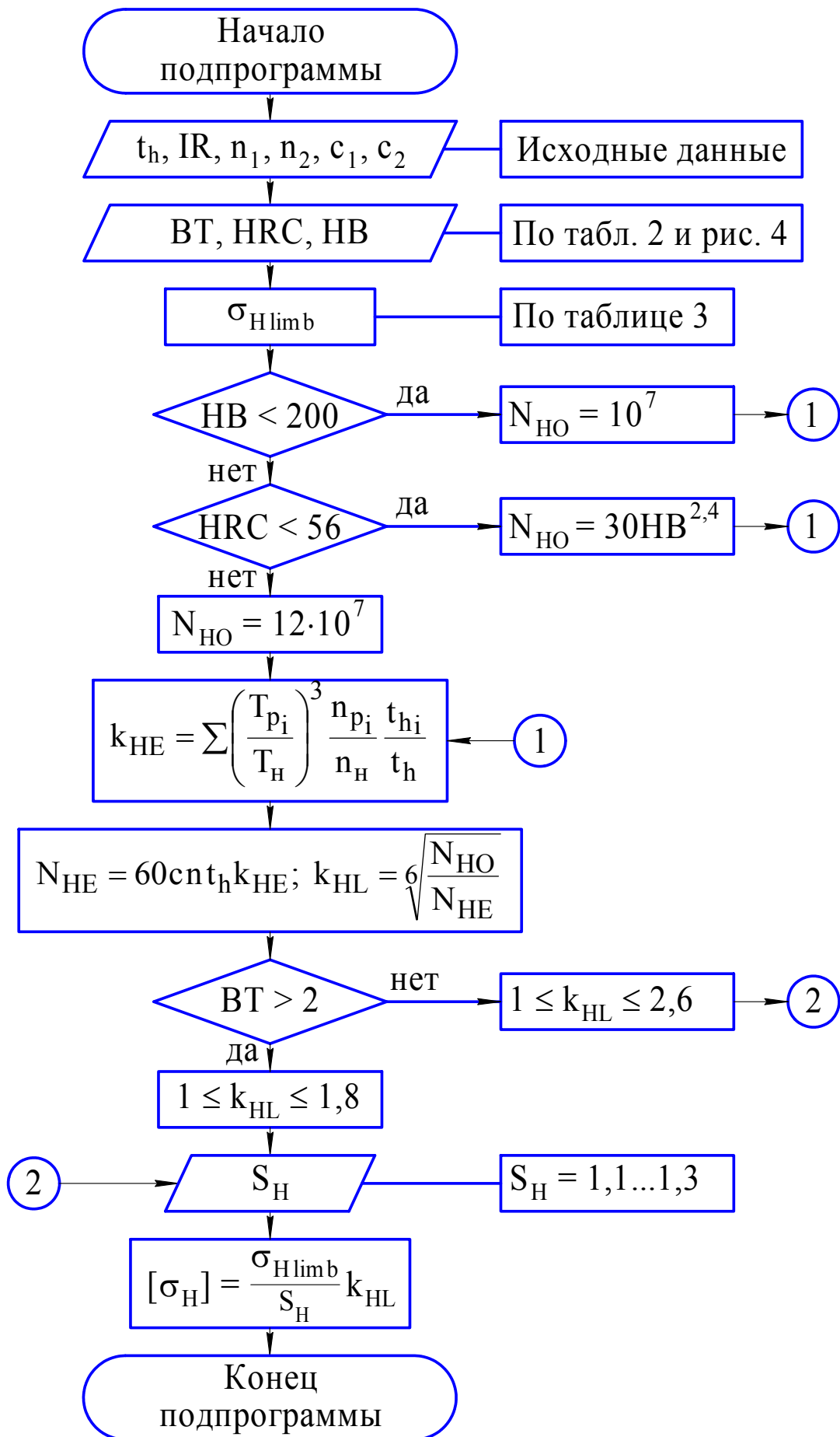
Рис. 3. Схема алгоритма определения допускаемых контактных напряжений
