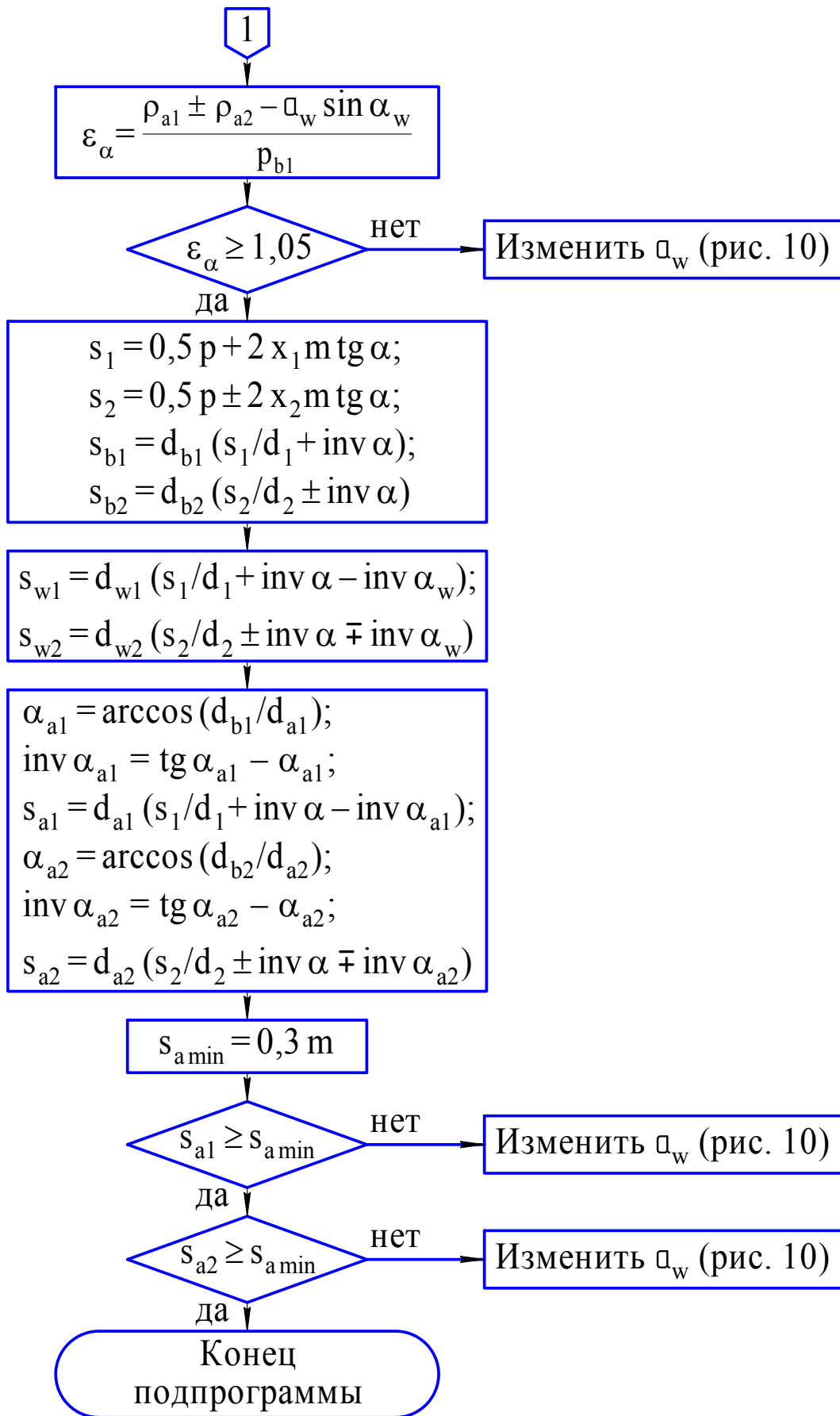
Рис. 13, б. Схема алгоритма геометрического расчёта передачи
