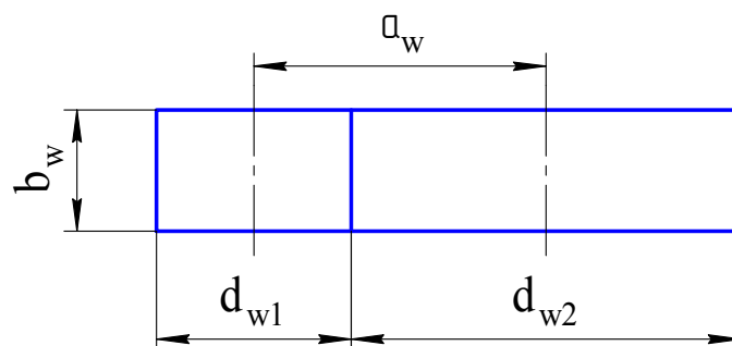
Рис. 8. Схема цилиндрической передачи
