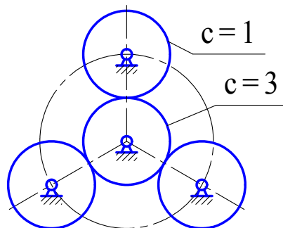
Рис. 6. Условия нагружения зуба
