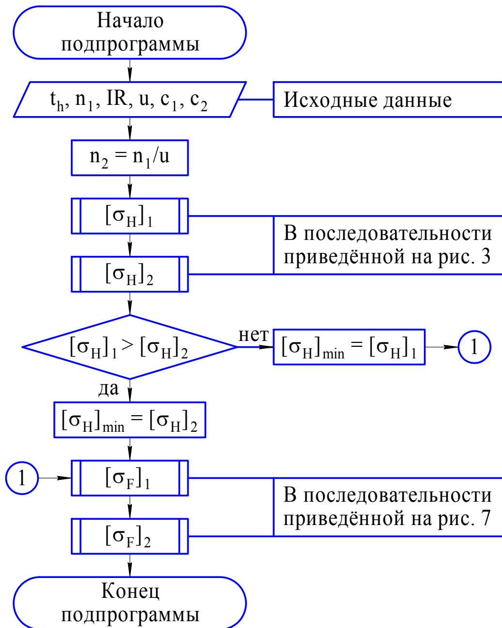
Рис. 2. Общая схема алгоритма определения допускаемых напряжений
