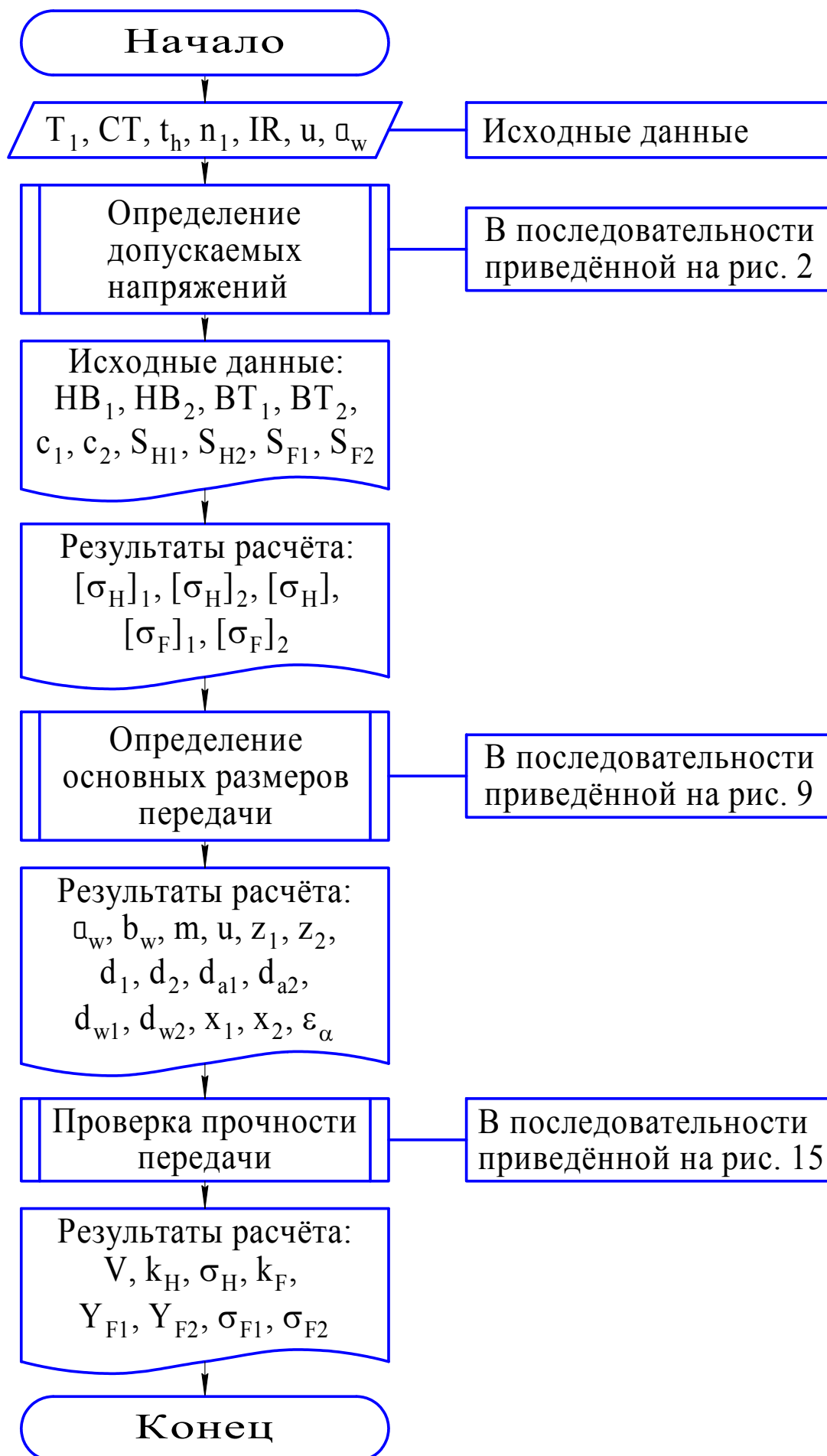
Рис. 1. Общая схема алгоритма расчёта цилиндрической передачи
