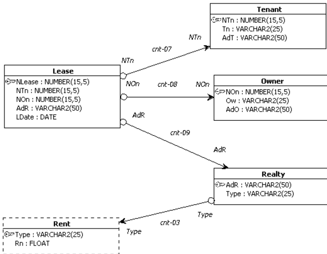
Рис. 2 Диаграмма базы данных «Аренда»
