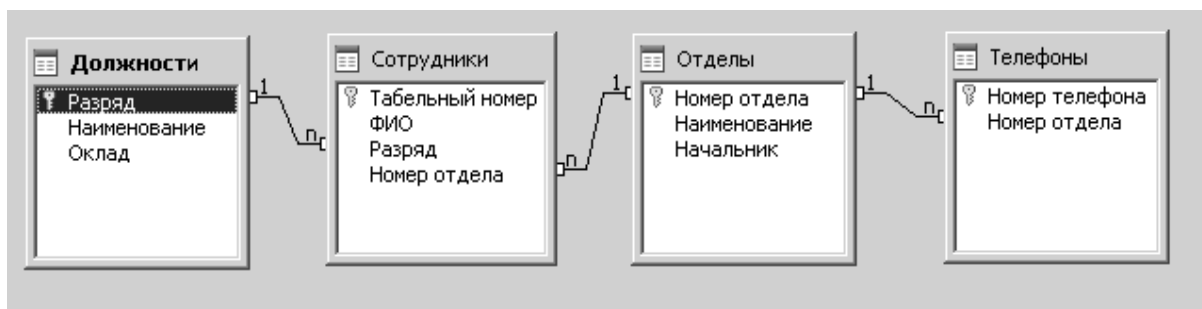
Рис. 1. Схема связей в БД «Фирма»
