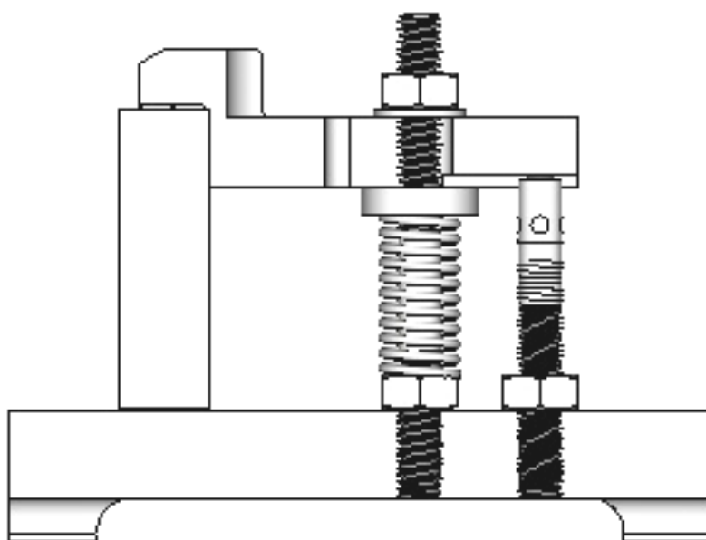
Рисунок 4.15. Конструкция зажимного устройства с прихватом ступенчатым
