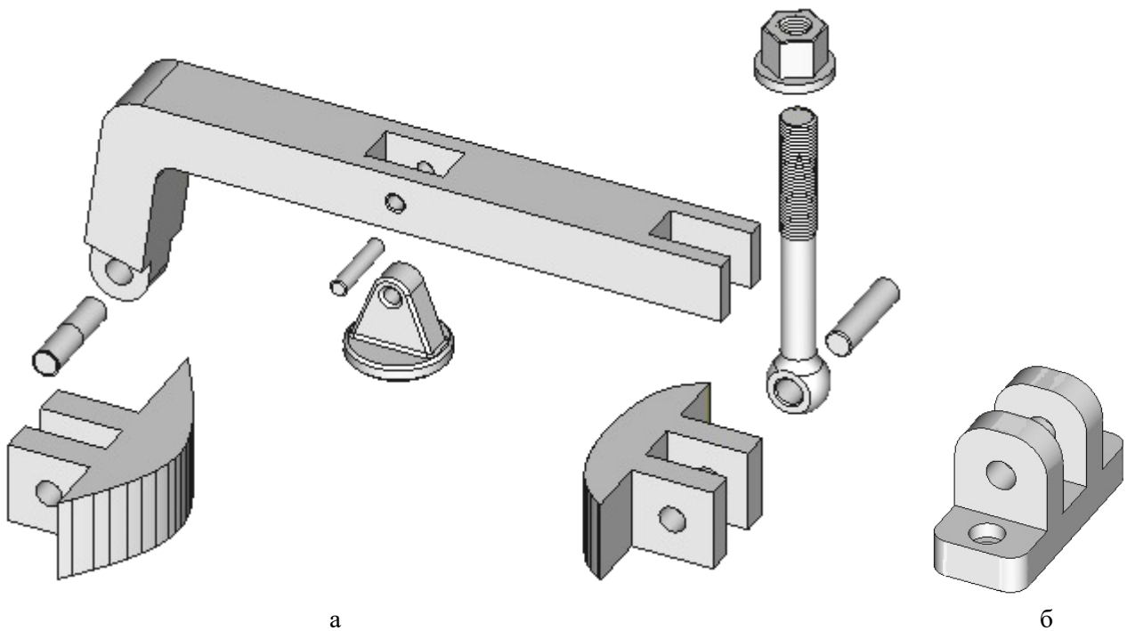
Рисунок 4.21. Устройство зажимного элемента: а – составные части и проушины основания (корпуса); б – вариант оформления проушин в виде кронштейна
