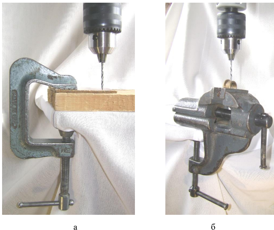
Рисунок 1.1. Сверление отверстия с применением бытовой дрели: а – фиксация заготовки в струбцине; б – фиксация заготовки в тисках
