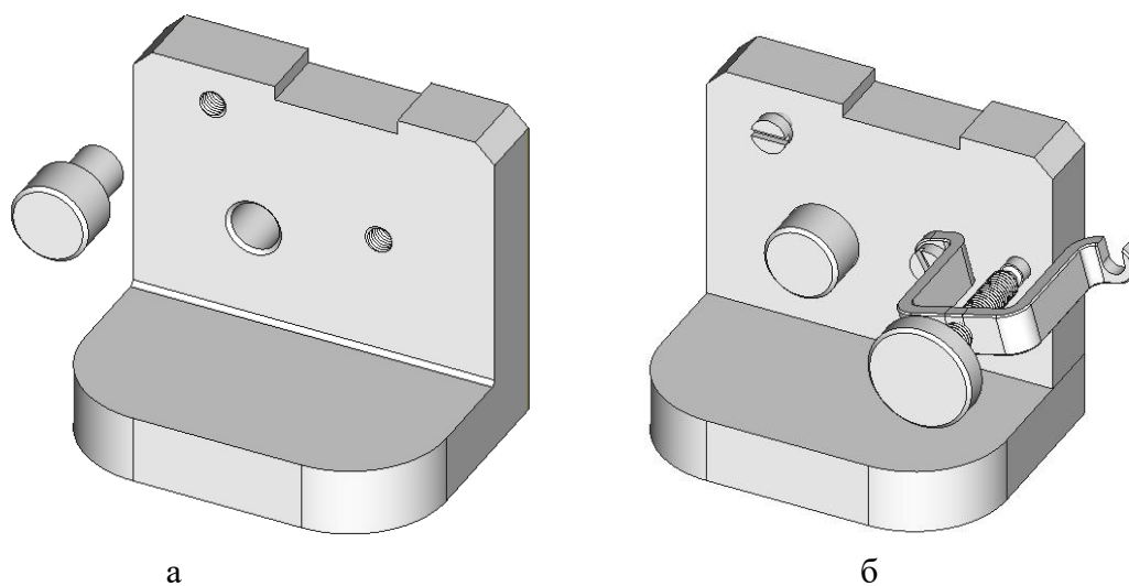
Рисунок 3.6. Приспособление с фигурным пазом и установочным пальцем: а – базовые детали; б - приспособление с зажимным элементом перед установкой
