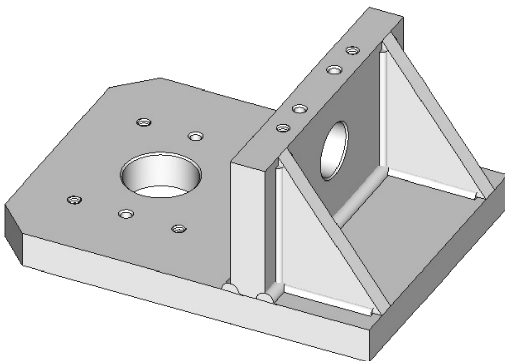
Рисунок 2.11. Корпус сварной
