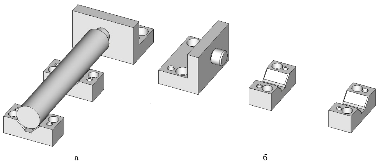
Рисунок 3.16. Цилиндрическая заготовка на призмах: а – положение заготовки; б – детали установочного элемента
