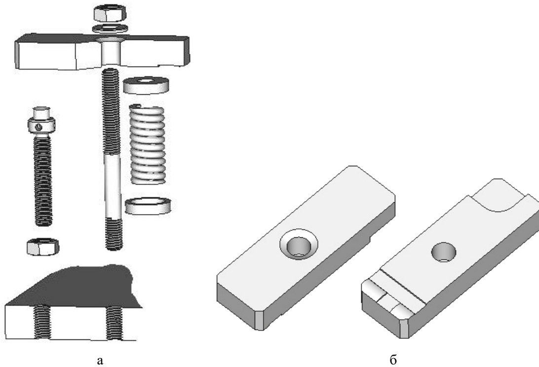
Рисунок 4.13. Детали зажимного устройства с прихватом прямым: а – составные части, слева направо и снизу вверх: контргайка; опора регулируемая; шпилька; чашка опорная нижняя; пружина; чашка опорная верхняя; прихват прямой; шайба; гайка; б – форма прихвата прямого (в альбоме [2] «поворотный»)
