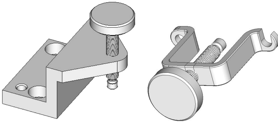
Рисунок 4.2. Установка нажимного винта в кронштейне и планке откидной
