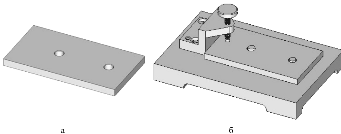
Рисунок 3.9. Установка заготовки «пластина» на пальцы: а – заготовка; б – заготовка в приспособлении перед обработкой
