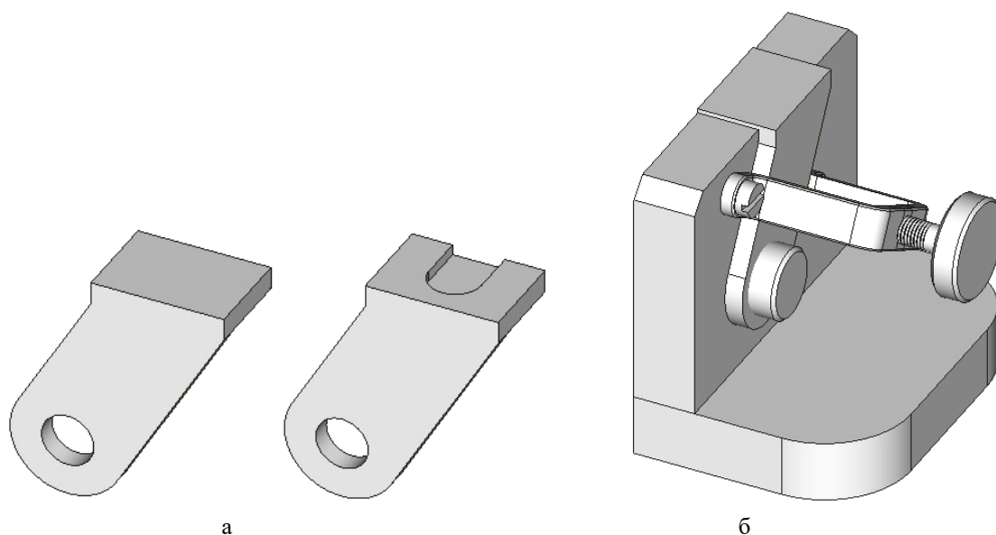
Рисунок 3.7. Установка заготовки в приспособление: а – заготовка до и после выполнения операции; б – заготовка в приспособлении
