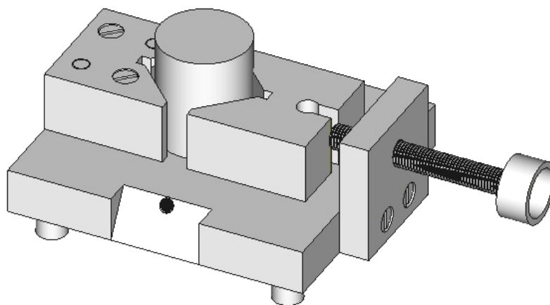
Рисунок 3.13. Установка заготовки с упором в неподвижную призму
