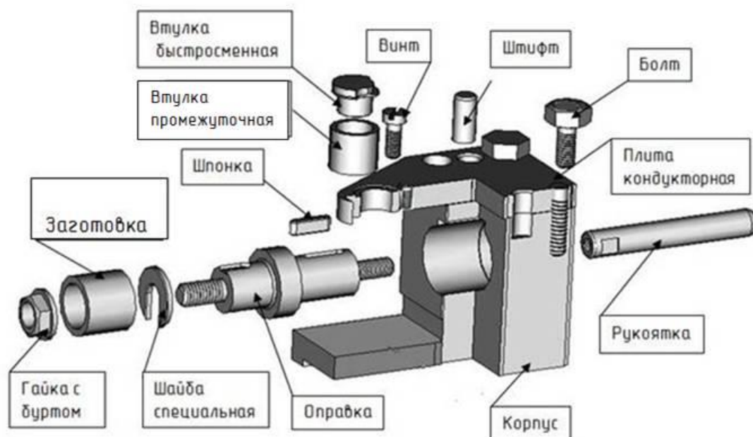
Рисунок 7.2. Устройство кондуктора
