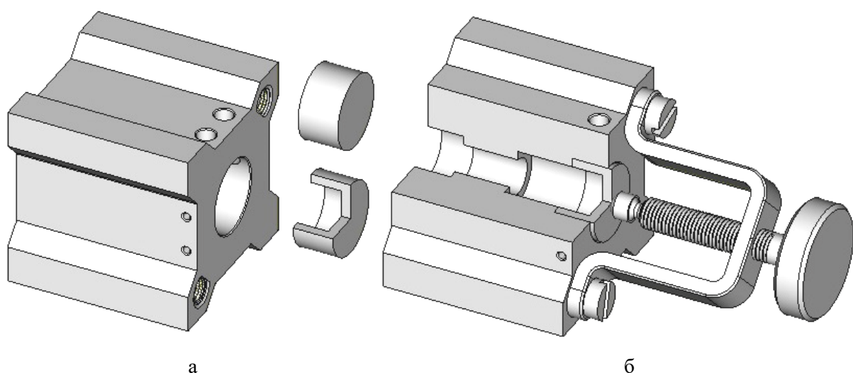
Рисунок 3.17. Установочный элемент – часть корпуса: а – корпус кантуемого кондуктора и заготовка; б - установка заготовки
