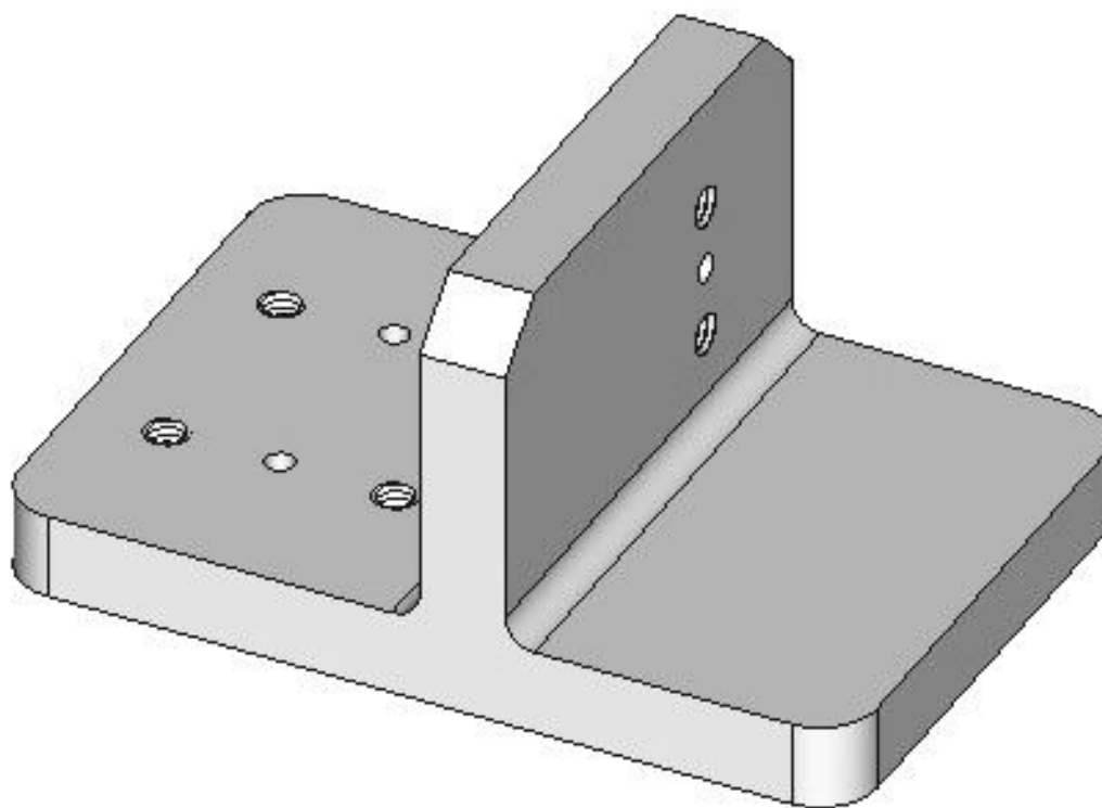
Рисунок 2.10. Вариант «Тавр» исполнения монолитного корпуса
