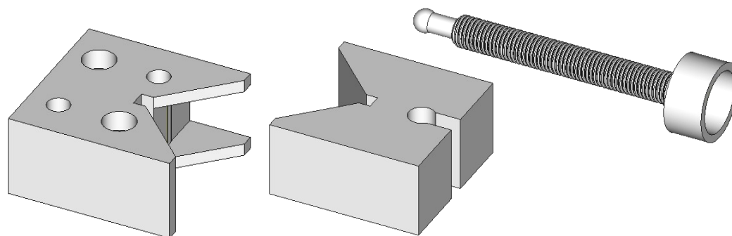
Рисунок 3.14. Детали установочного элемента: неподвижная призма, подвижная призма, винт
