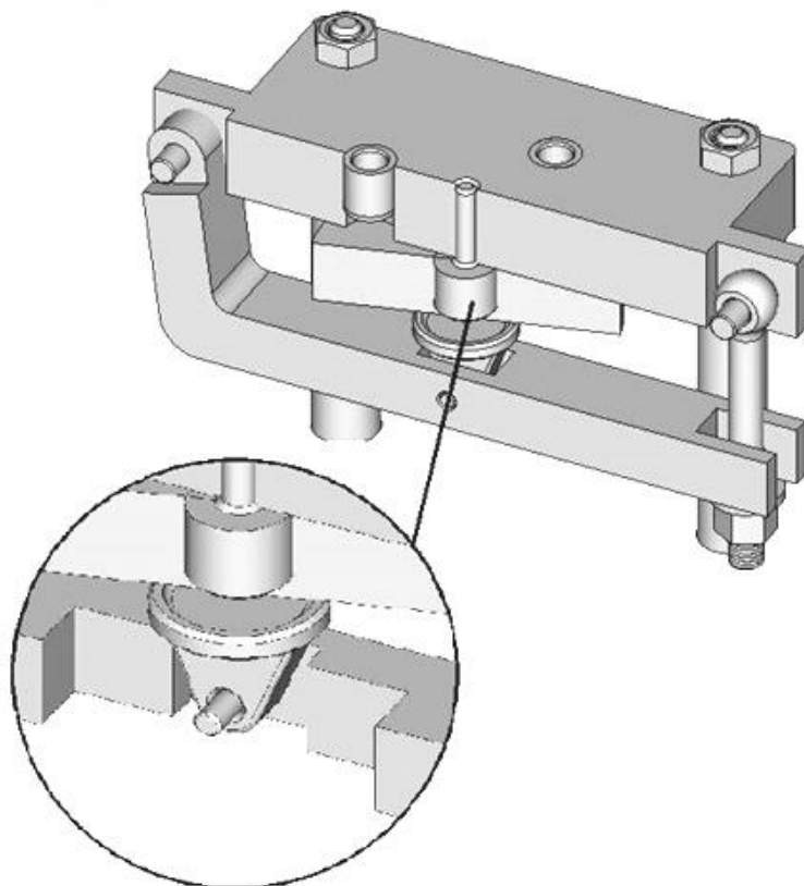
Рисунок 4.20. Схема работы зажимного устройства
