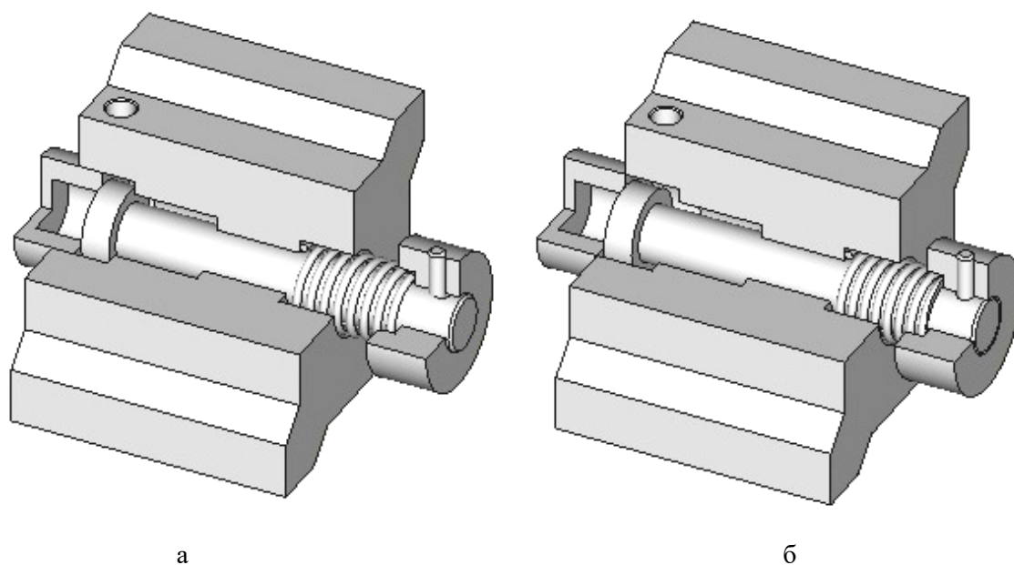
3.19. Работа выталкивающего устройства: а – начало демонтажа; б - завершение демонтажа
