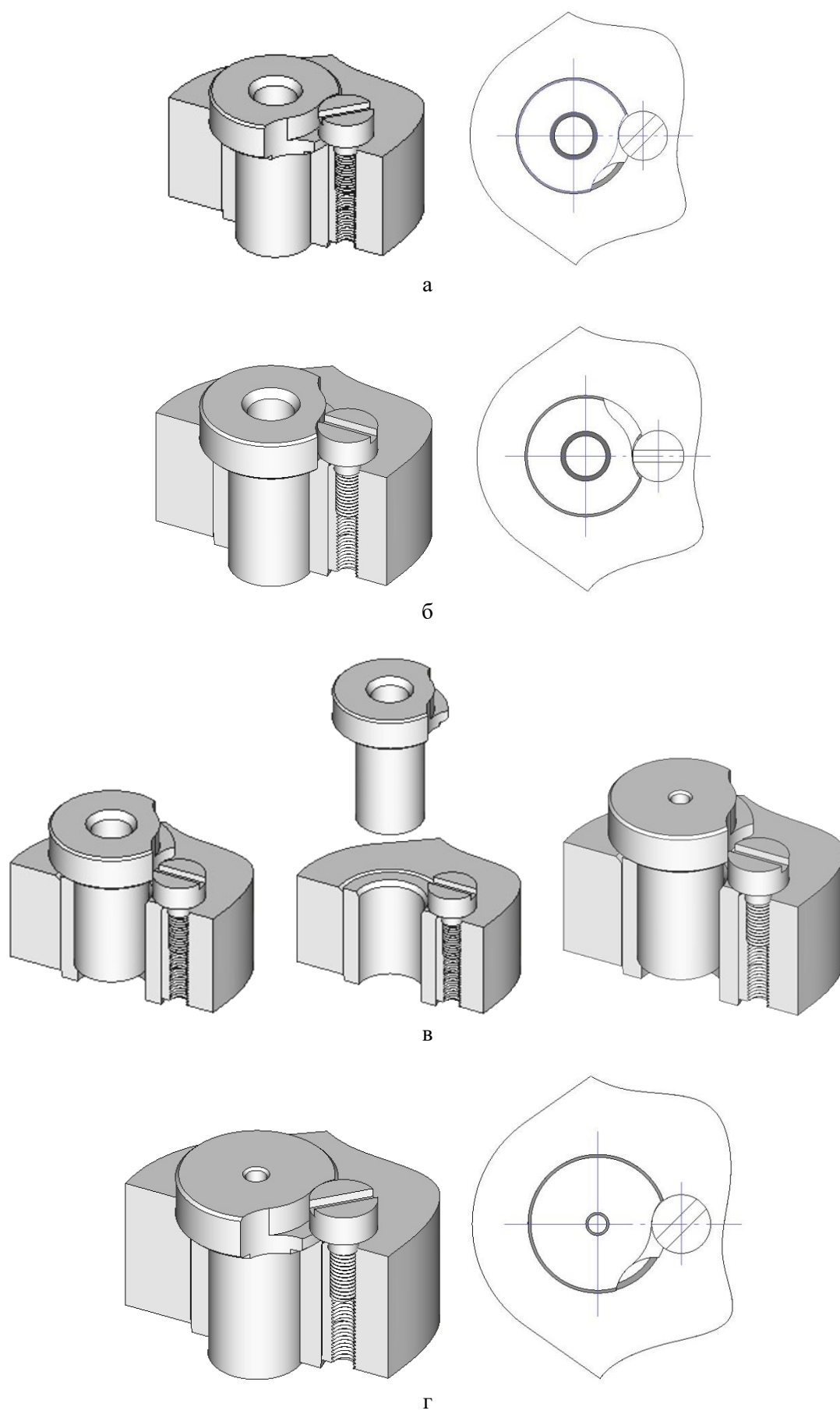
Рисунок 5.5. Этапы замены быстросменной втулки
