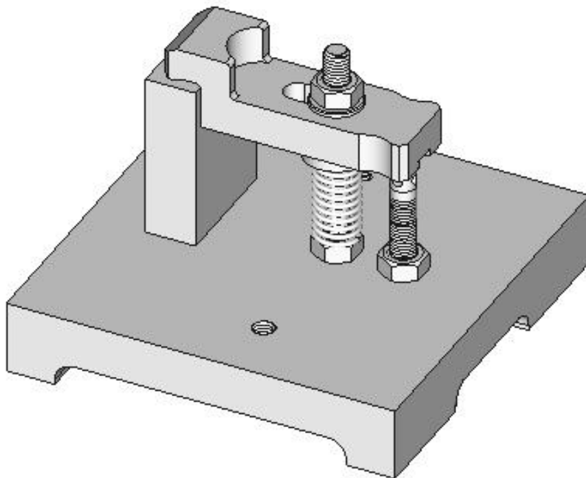
Рисунок 4.14. Прихват ступенчатый в приспособлении с заготовкой
