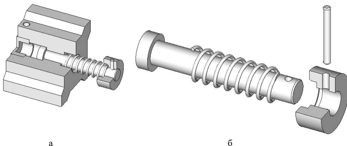
Рисунок 3.18. Конструкция выталкивающего устройства: а – рабочее положение кондуктора; б – детали устройства
