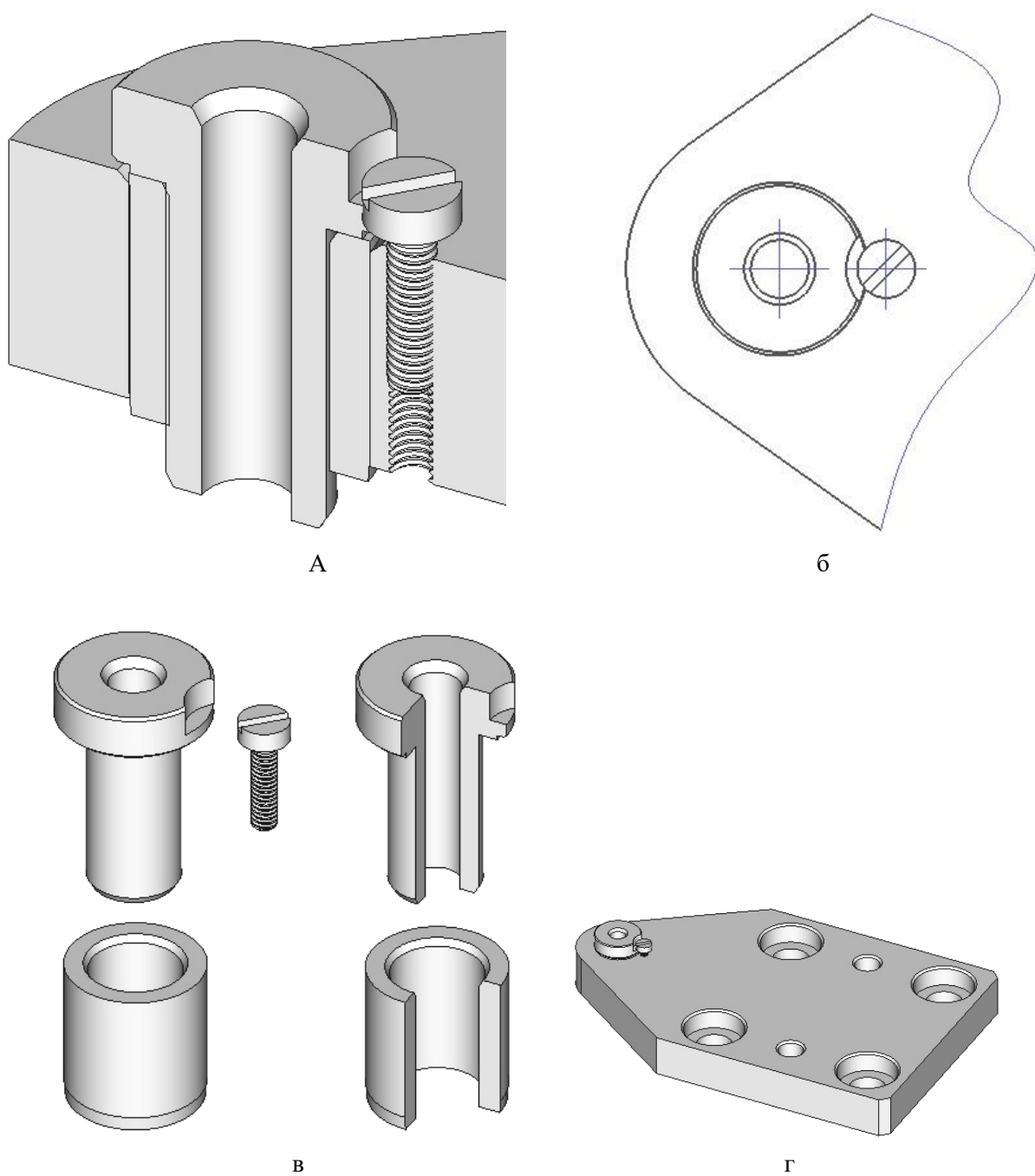
Рисунок 5.3. Втулка кондукторная сменная: а – втулка сменная установлена в кондукторную плиту через промежуточную втулку и зафиксирована винтом; б – вид сверху соединения деталей; в – втулка кондукторная сменная, втулка промежуточная, винт; г – положение втулок на кондукторной плите
