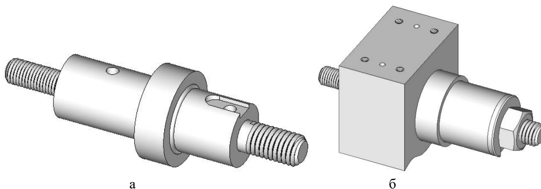
Рисунок 3.10. Горизонтальная оправка для заготовки «труба / втулка»: а – оправка отдельно; б – оправка в корпусе кондуктора
