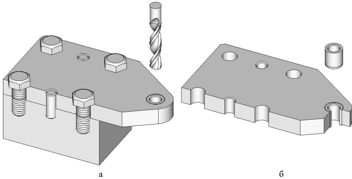
Рисунок 5.1. Втулка кондукторная постоянная в плите кондукторной: а – вариант установки кондукторной плиты на корпусе; б – установка втулки кондукторной постоянной в плите
