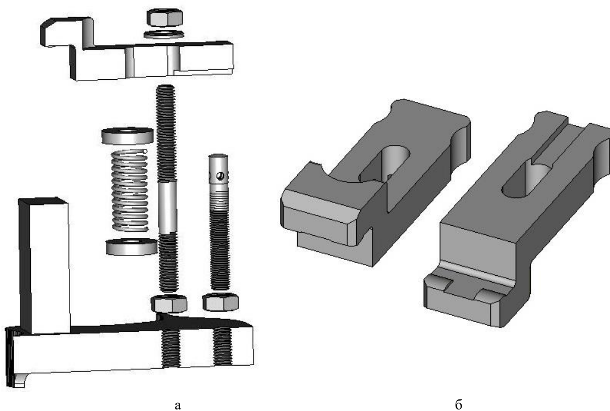
Рисунок 4.16. Детали зажимного устройства с прихватом ступенчатым: а – составные части, слева направо и снизу вверх: чашка опорная нижняя; пружина; чашка опорная верхняя; контргайка; шпилька; прихват ступенчатый; шайба; гайка; контргайка; опора регулируемая; б – форма прихвата прямого (в альбоме [2] «поворотный»)
