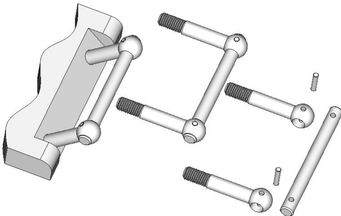
Рисунок 2.15. Рукоятка сборная
