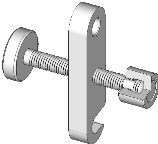
Рисунок 4.3. Подвижное соединение пяты и винта в проточке
