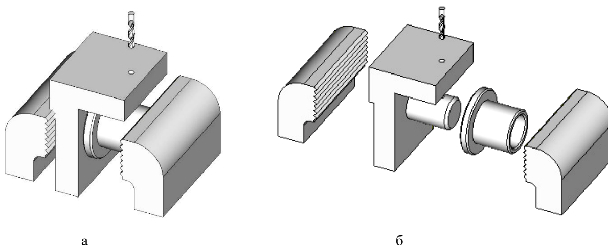
Рисунок 1.2. Вариант конструкции приспособления для сверления в тисках: а – приспособление в сборе; б – детали рассыпью
