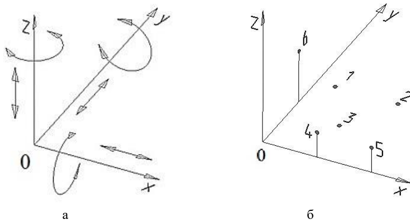
Рисунок 3.1. Схема базирования по «правилу 6 точек»: а – возможные движения; б – комплект точек, исключаящий движение
