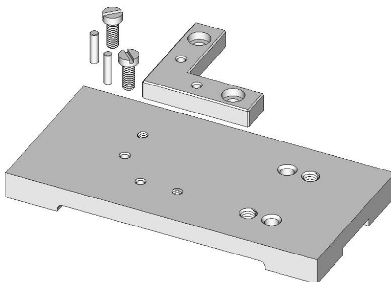
Рисунок 3.5. Монтаж уголка на основании
