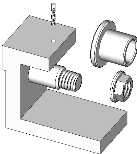
Рисунок 1.3. Универсальный вариант конструкции кондуктора
