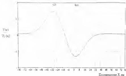
Рис. 1 Позиционные характеристики экспериментальной U и аппроксимирующей W(a, b, c, x_0) функции при a=0,12 , b=2,037 \cdot 10^{-3} , c=0,218 , x_0 = -12,591
